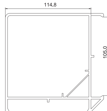
P8059 90°拼接材
