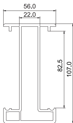
P6058 180°拼接材
