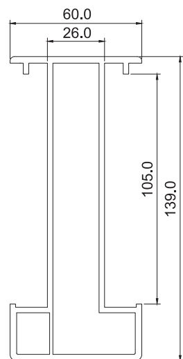
P905B 180°拼接材
