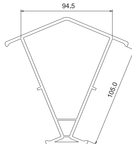
P8054 45°拼接材
