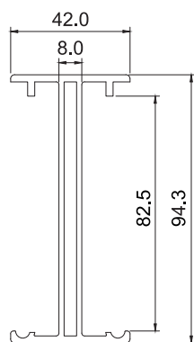
P6055 180°拼接材
