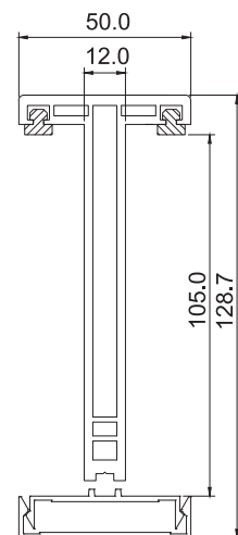
P905T 180°T拼接材
