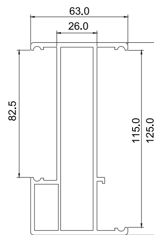
P6759 180°併列材
