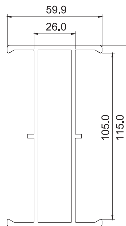
P8058 180°拼接材
