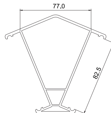
P6054 45°拼接材
