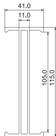
P9058 180°拼接材
