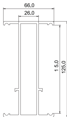
P6758 180°拼接材
