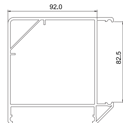
P6059 90°拼接材
