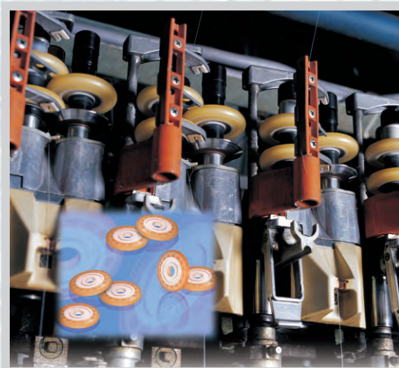
PU 磨擦胎 PU Friction DISC
