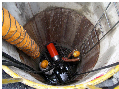
PVC推進管
