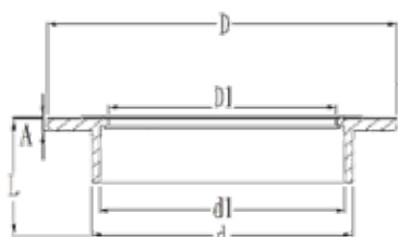
管固定座 Beam Fittings
