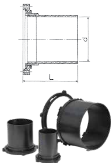
組合式穿樑接頭 Assembly type Beam Fittings 單位：mm
