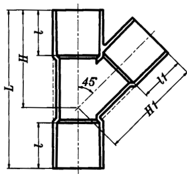
45° Y型接頭 45° Wye
