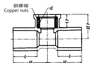
龍 T 入銅接頭 Faucet Fitting - Fixture TEE 單位: mm
