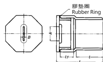
清除孔接頭 Cleanout Bushing
