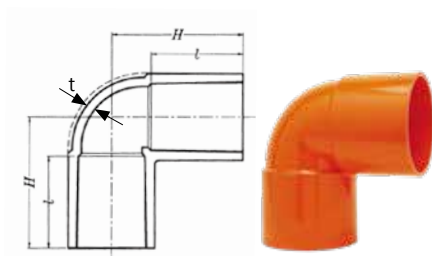
90° L 型接頭 90° Elbow 單位: mm
