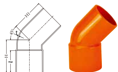
45° L型單放口接頭 45° Elbow With Spigot End 單位: mm
