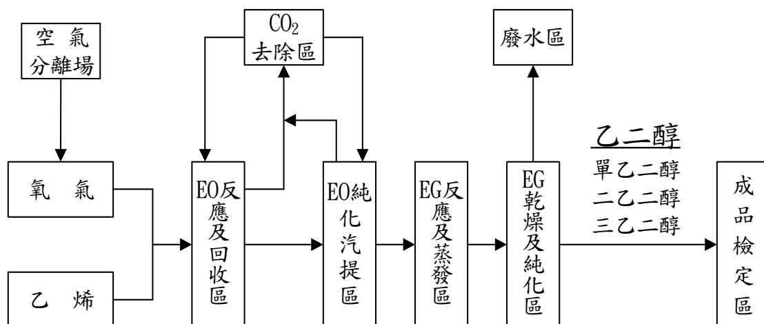
乙二醇生產流程圖
