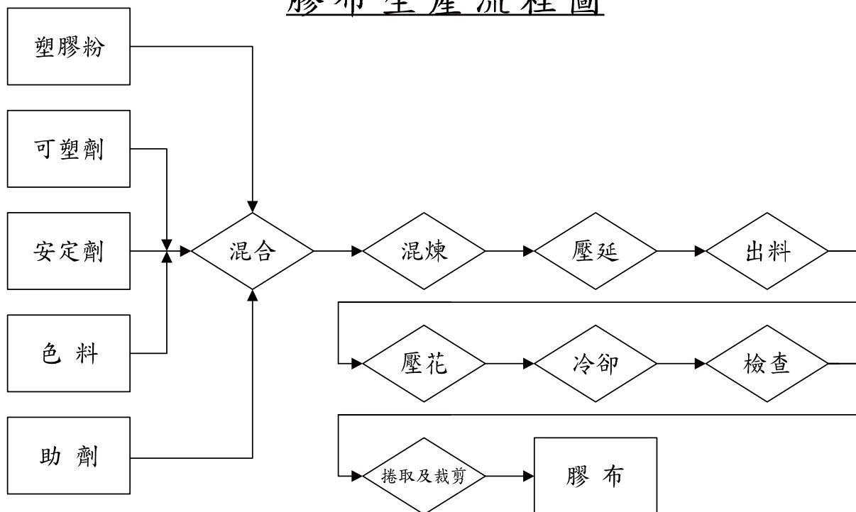
膠布生產流程圖
