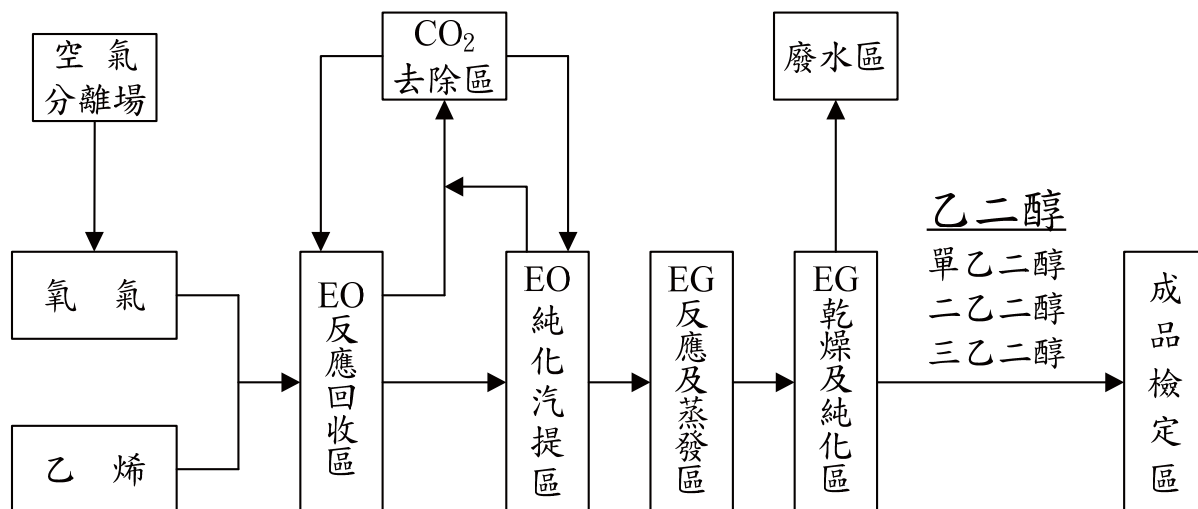
乙二醇生產流程圖
